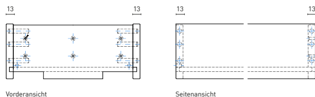
Vorderansicht
