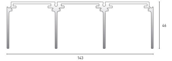
Deckenschiene dreiläufig
