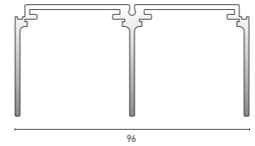
Deckenschiene zweiläufig
