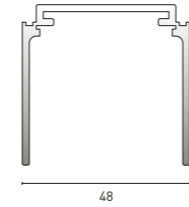
Deckenschiene einläufig
